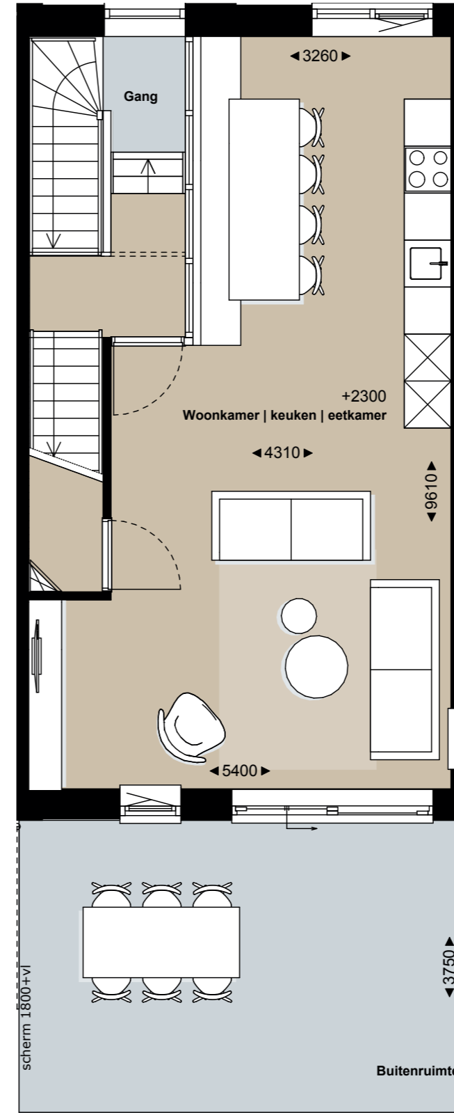
⇧ VERDIEPING 1
