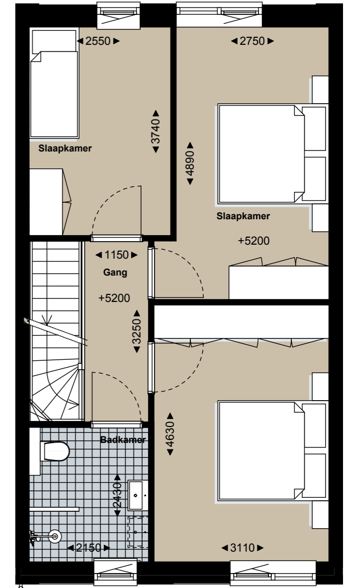
⇧ VERDIEPING 2
